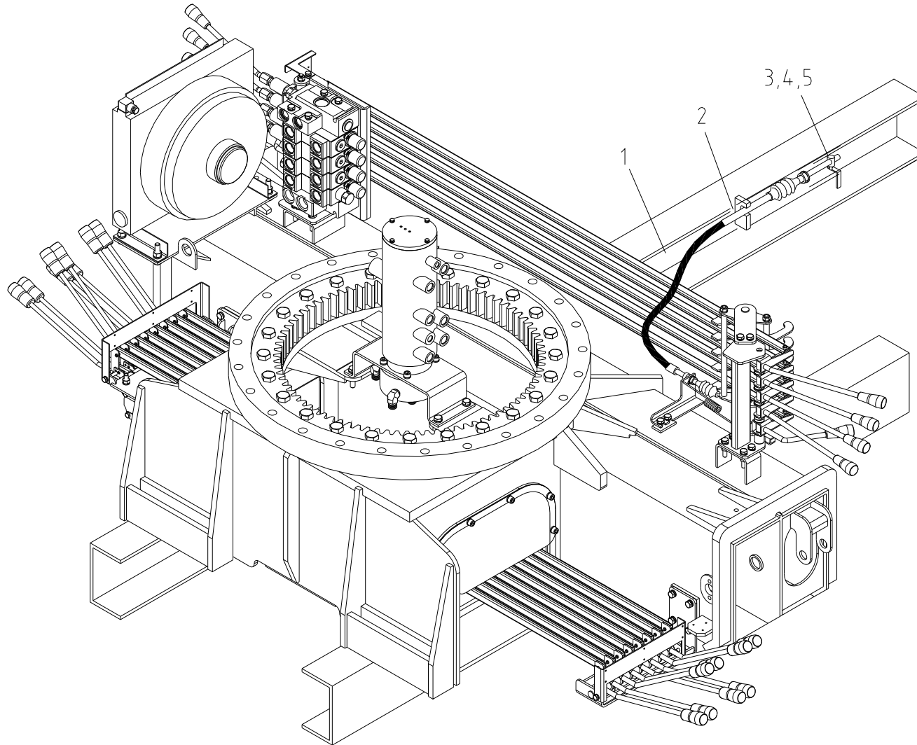
악셀 시스템 파트 Fig. 8-3 SCS1015 ACC'L SYSTEM PART
