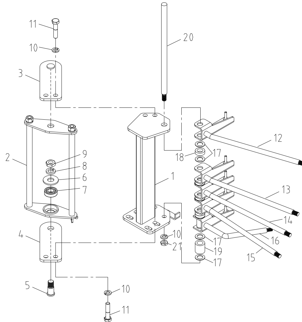
레버 스텐드 셋 Fig. 3-3-2 SCS1015 LEVER STAND SET
