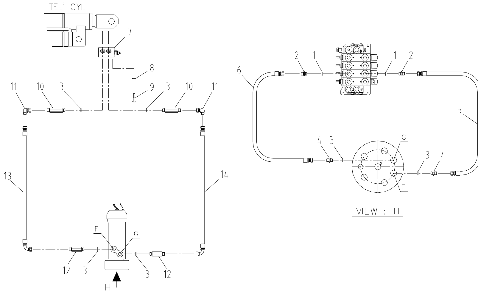
텔레스코픽 배관 Fig. 5-4 SCS1015 TELESCOPIC PIPING
