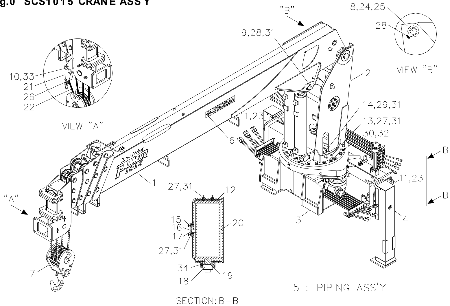
크레인 조립체 Fig.0 SCS1015 CRANE ASS'Y
