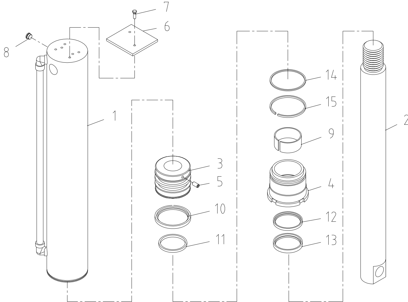
잭 실린더 조립체 Fig. 4-2 SCS1015 JACK CYL' ASS'Y
