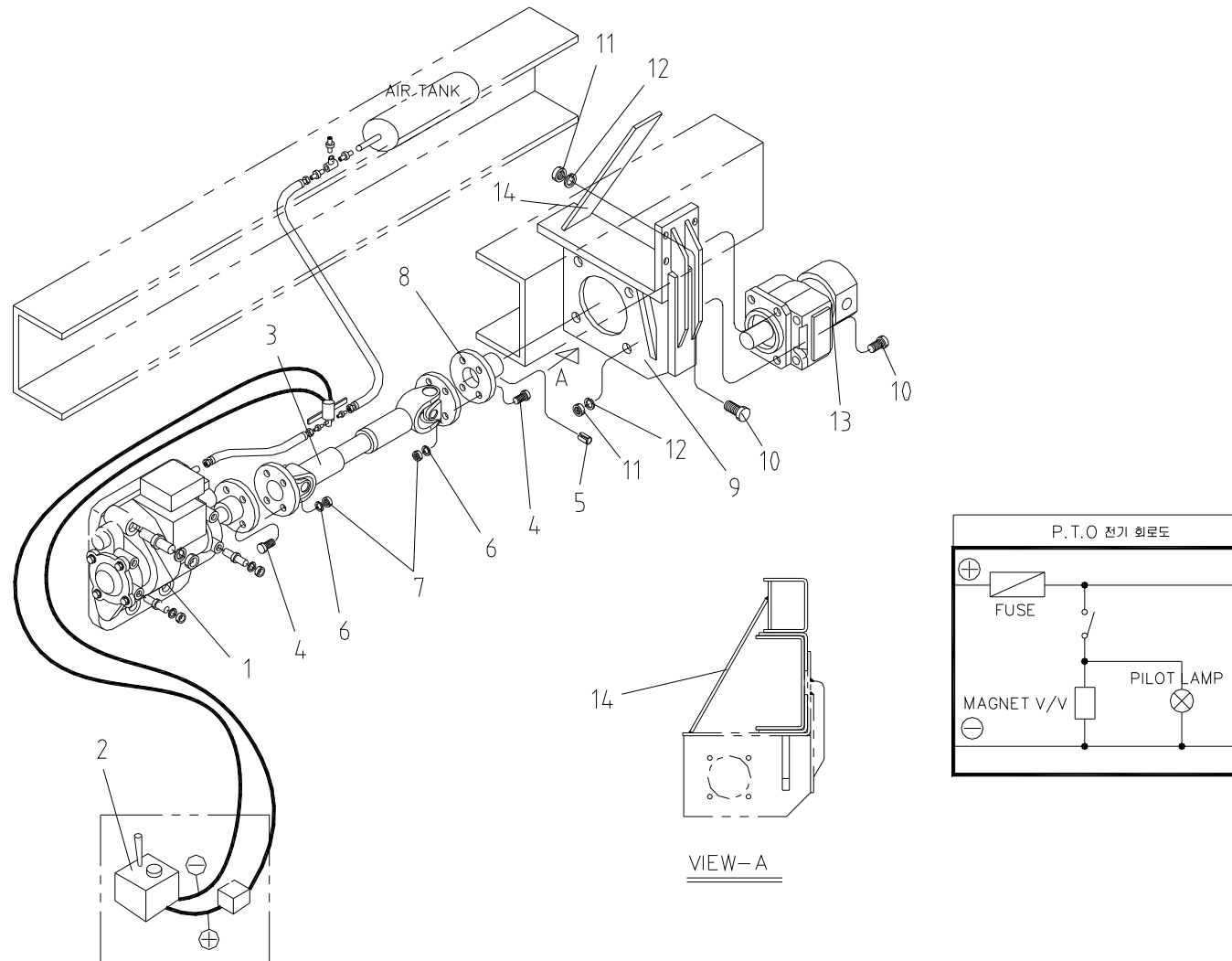
P.T.O & 펌프 파트 Fig. 8-1 SCS1015 P.T.O & PUMP PART
