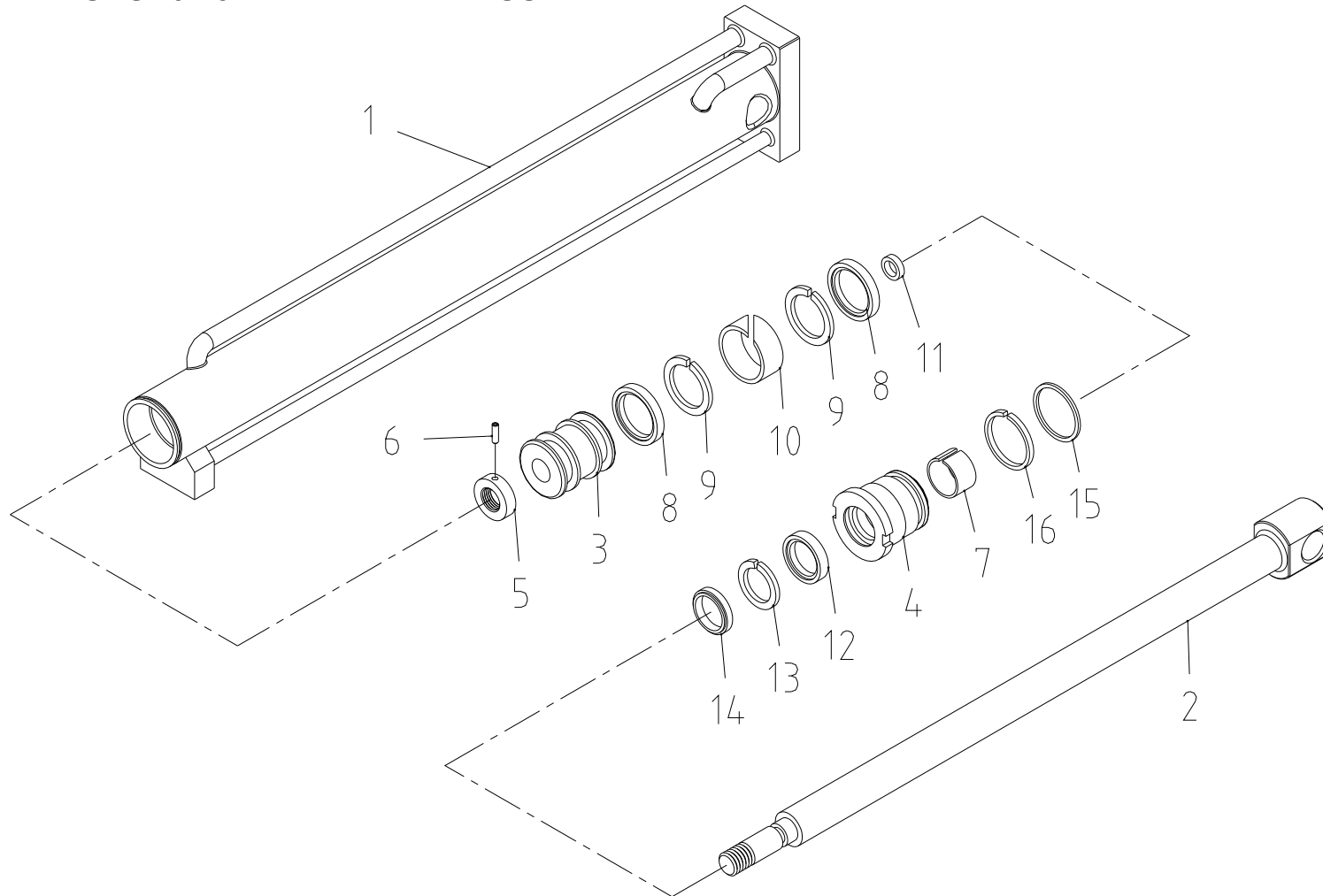
익스펜드 실린더 조립체 Fig. 4-1 SCS1015 EXPAND CYL' ASS'Y
