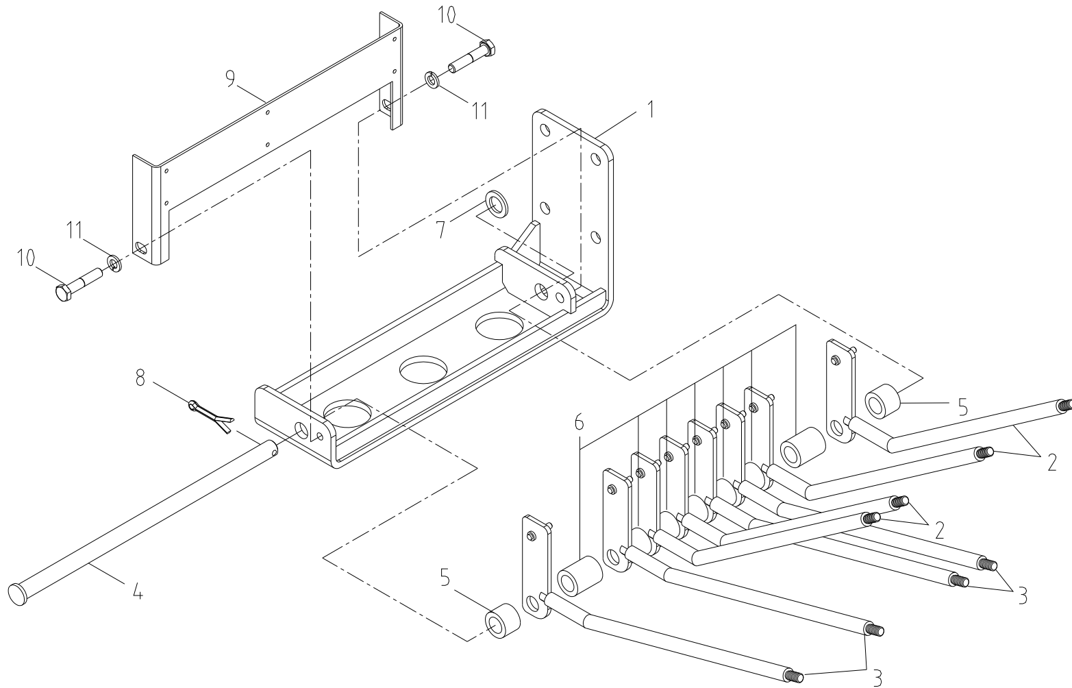
레버 스텐드 셋 Fig. 3-4-2 SCS1015 LEVER STAND SET
