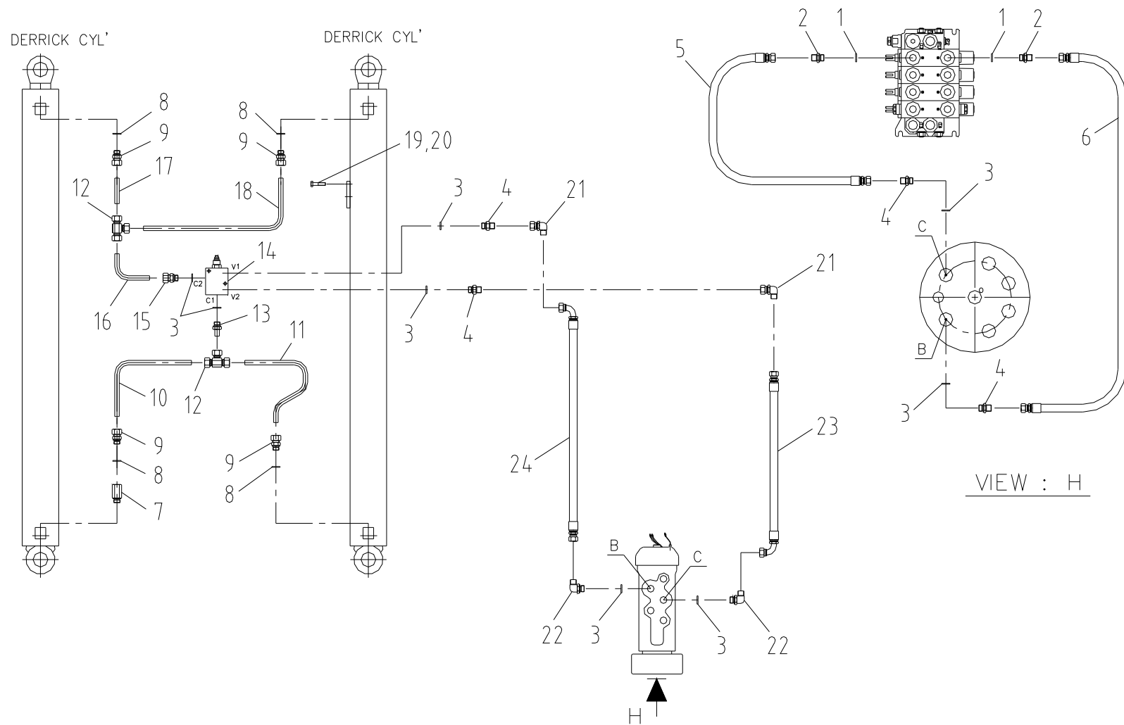
데릭 배관 Fig. 5-2 SCS1015 DERRICK PIPING
