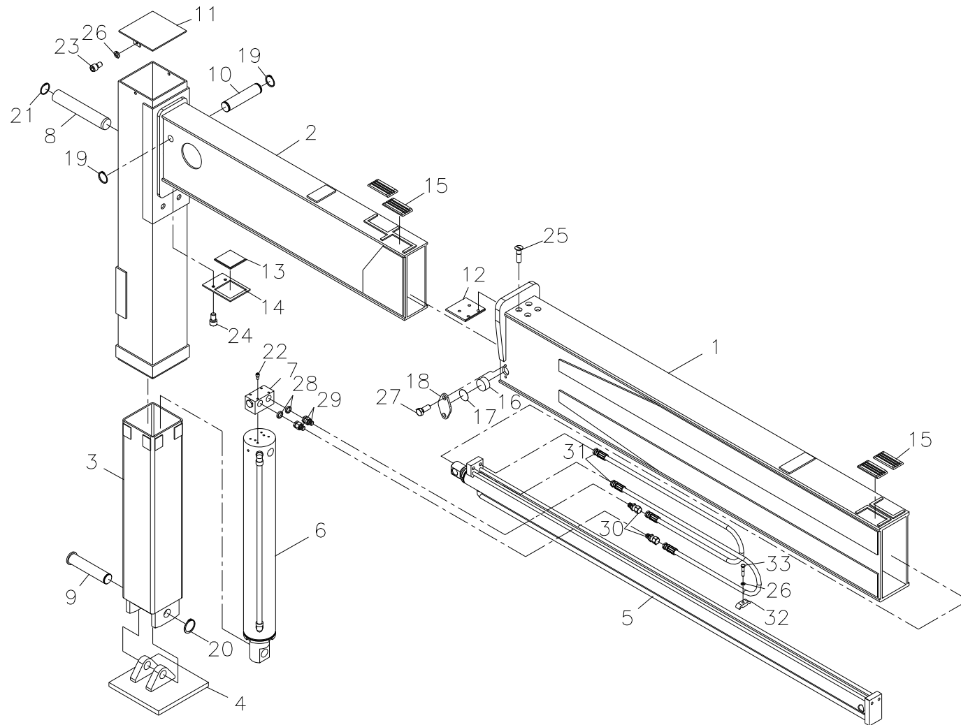
아우트리거 조립체 Fig. 4 SCS1015 OUTRIGGER ASS'Y
