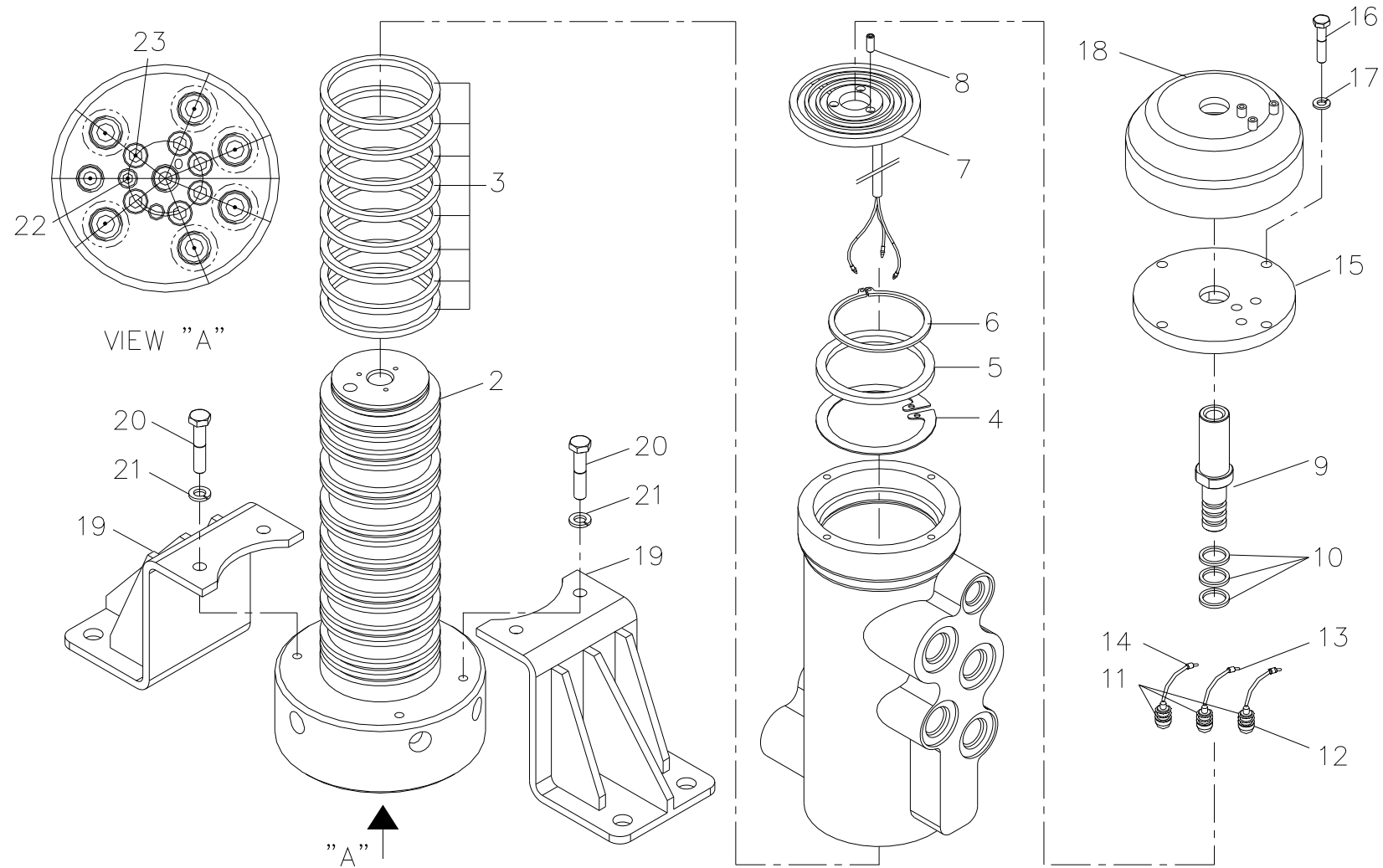
로타리 조인트 조립체 Fig. 3-2 SCS1015 ROTARY JOINT ASS'Y
