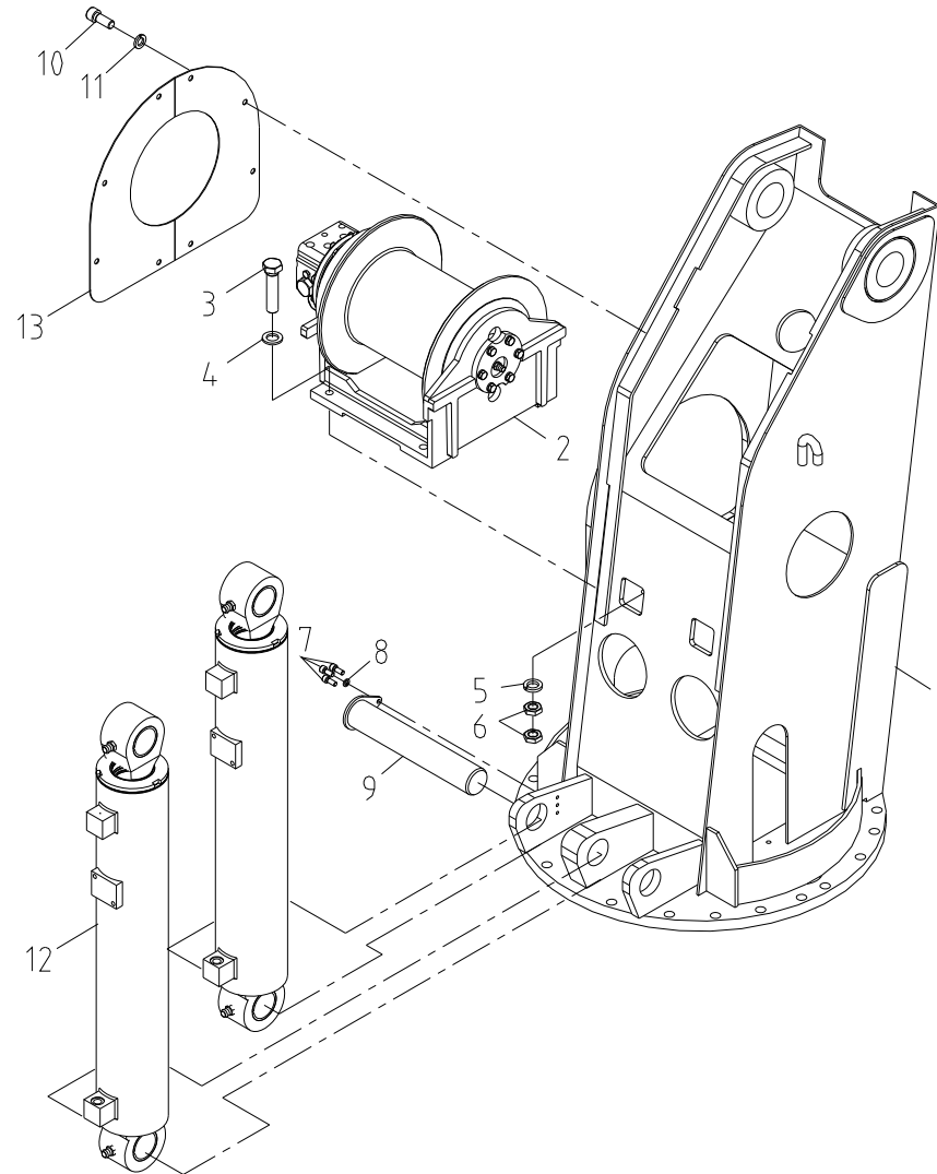
스윙 포스트 조립체 Fig. 2 SCS1015 SWING POST ASS'Y
