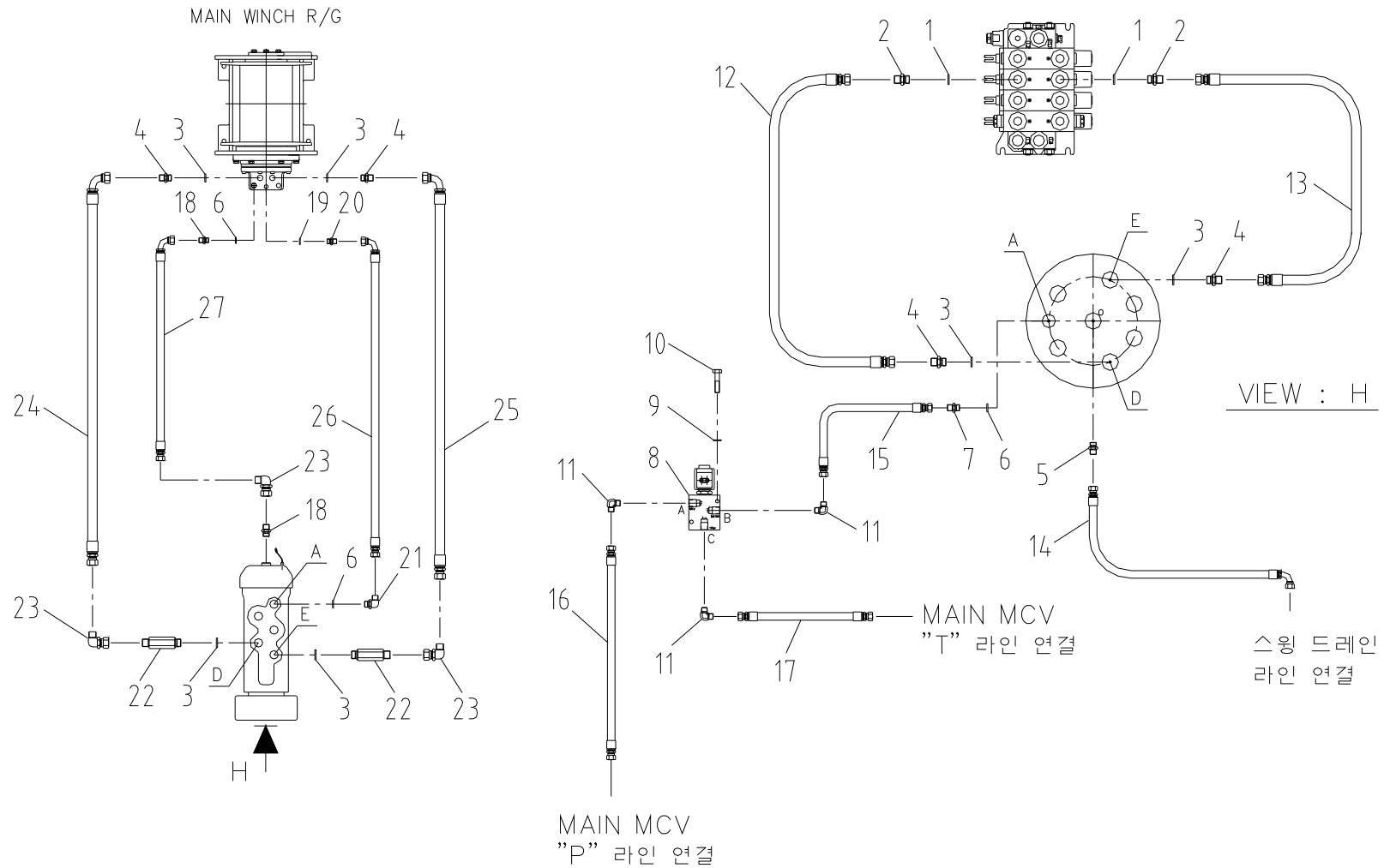
원치 배관 Fig. 5-3 SCS1015 WINCH PIPING
