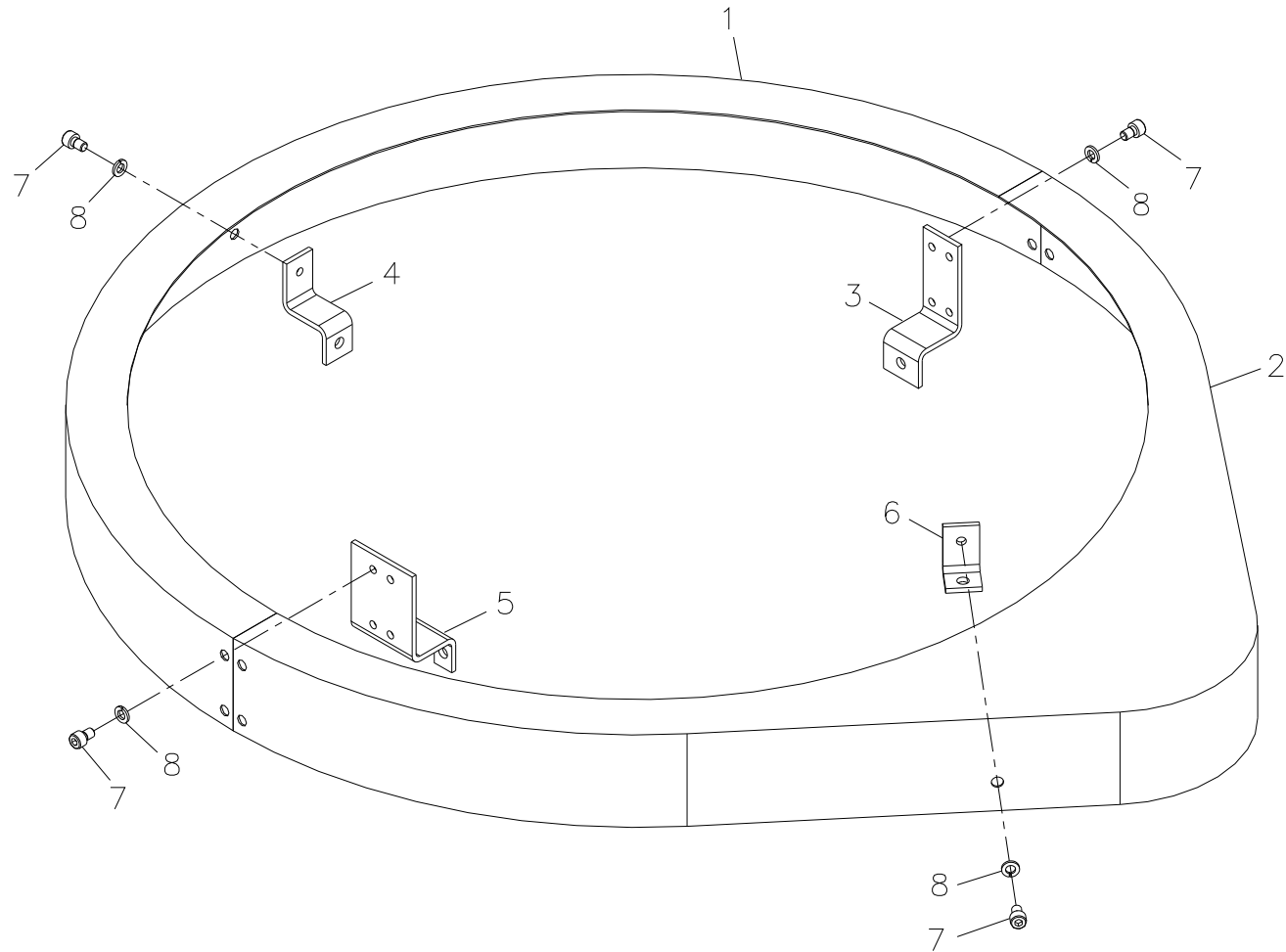
스윙 기어 커버 Fig. 3-5 SCS1015 SWING GEAR COVER
