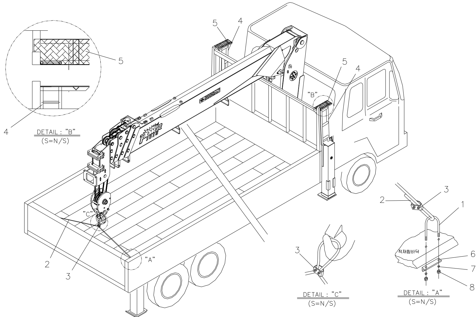
로딩 박스 파트 Fig. 8-5 SCS1015 LOADING BOX PART
