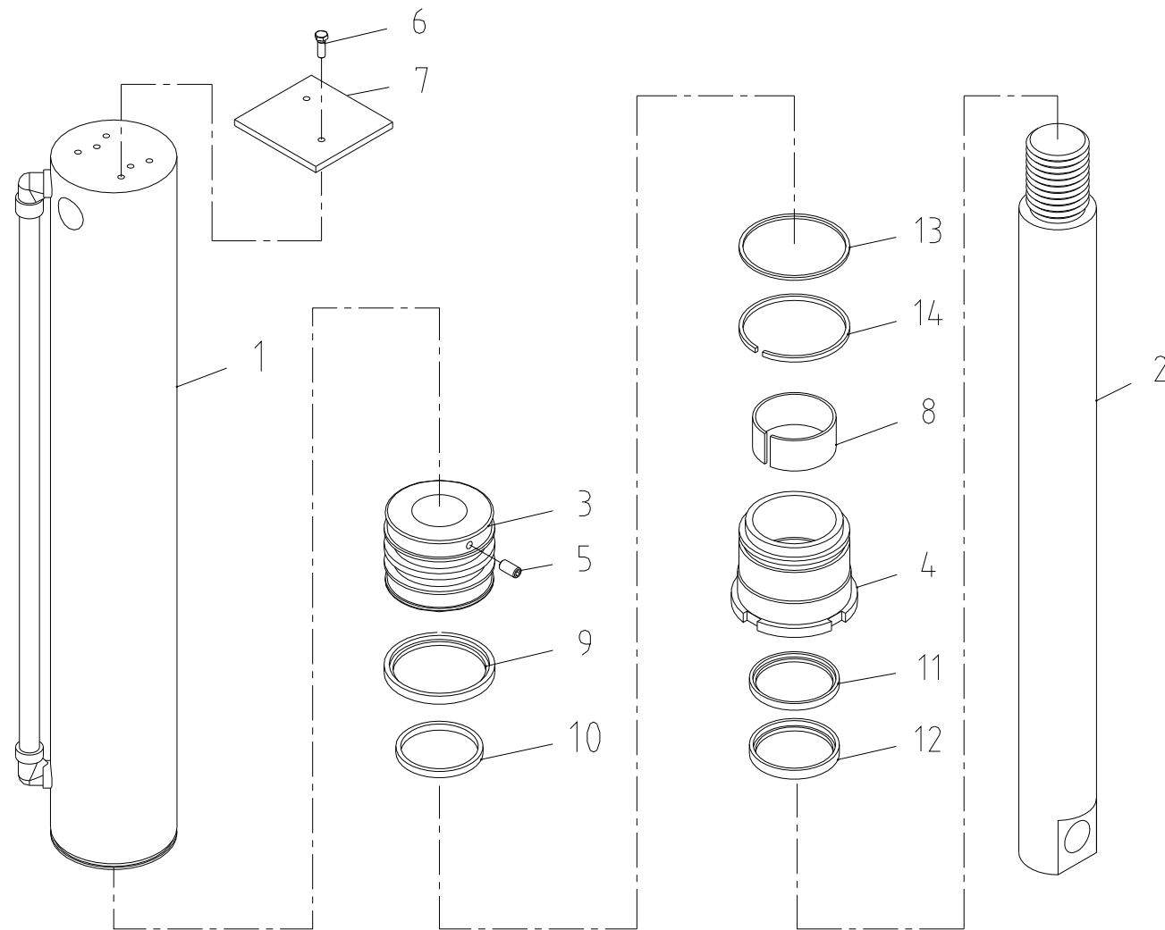
잭 실린더 조립체 Fig. 8-2-1-1 SCS1015 JACK CYL' ASS'Y
